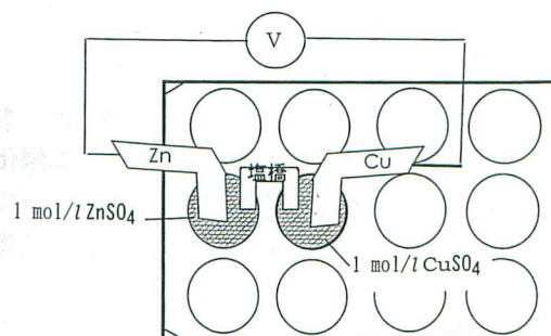
図2 ろ紙片の塩橋を使ったダニエル電池。
